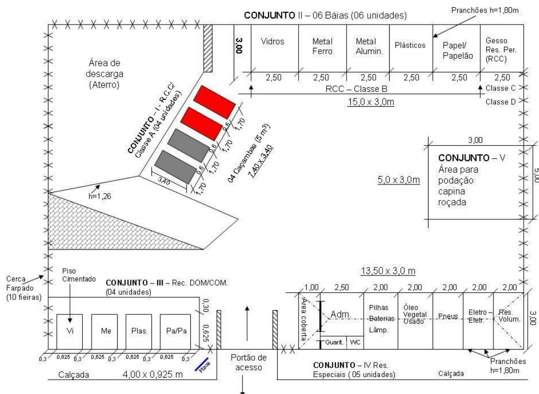
Figura 69 - Proposta de planta de ECOPONTO Fonte: SERENCO, 2.012.
